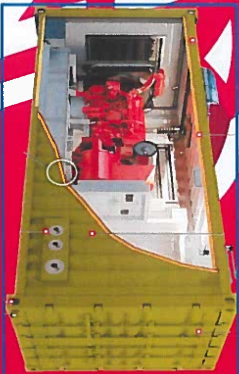
Дизельный генератор АД-40
